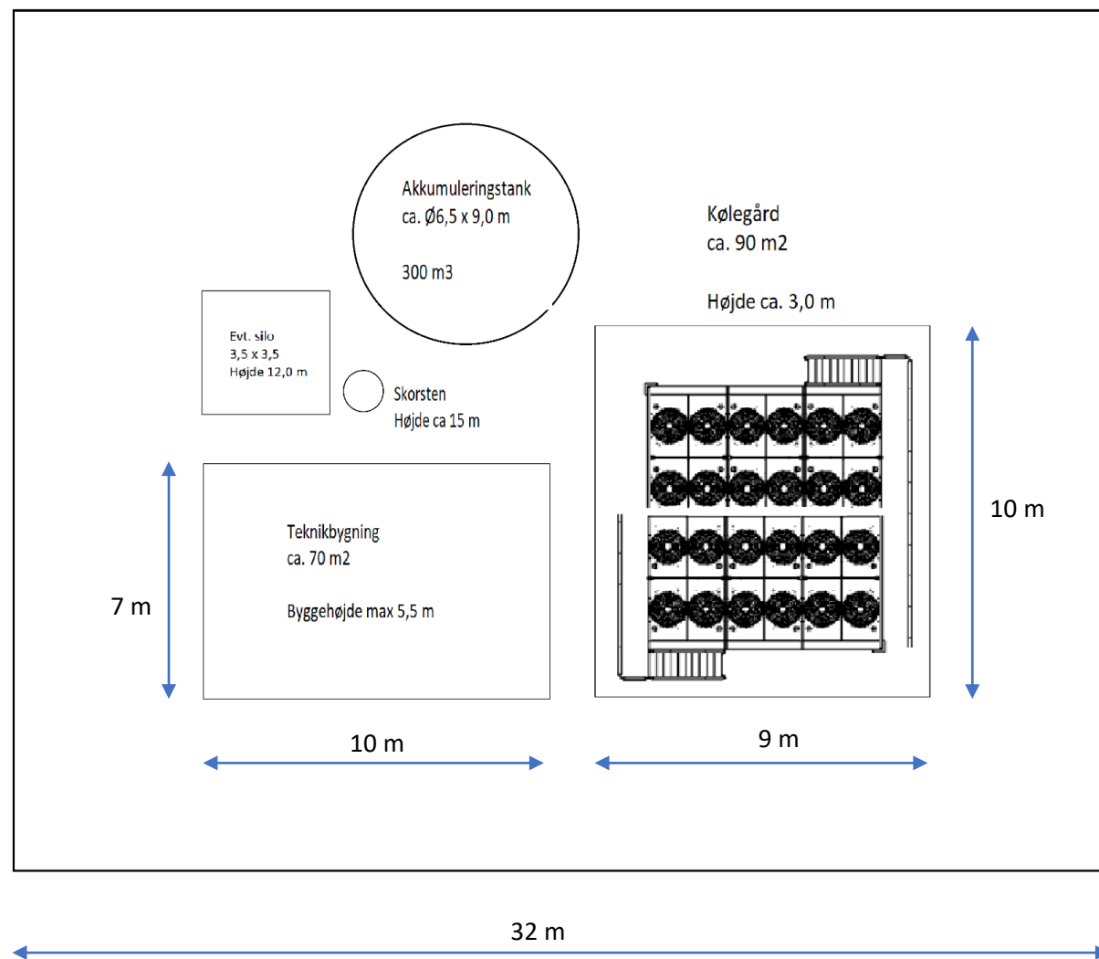
Grundplan med areal på 25 x 32 m
